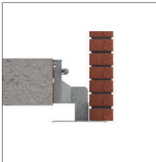
Spouwafsluiting met T-profiel
